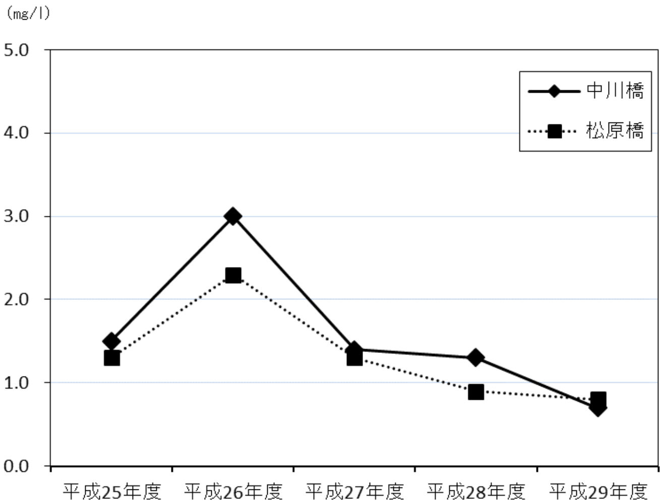
図 8 河川水質調査結果（BOD）－中川（類型指定なし）－
