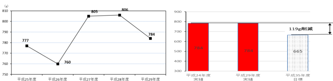
図 11 1 人 1 日あたりのごみ処理量の推移と目標値
