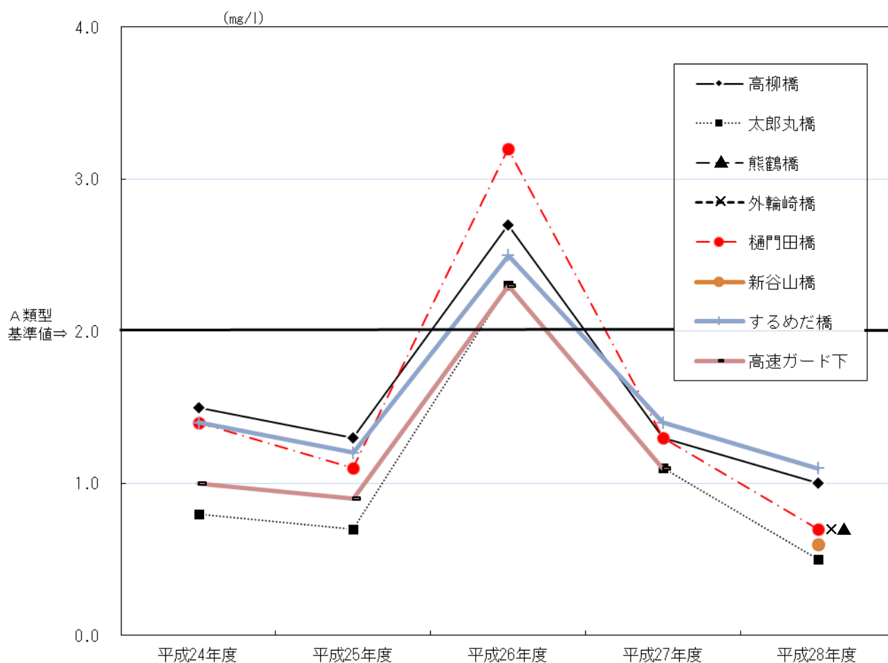
図 7 河川水質（BOD）調査結果の推移—大根川水系（A 類型）—
