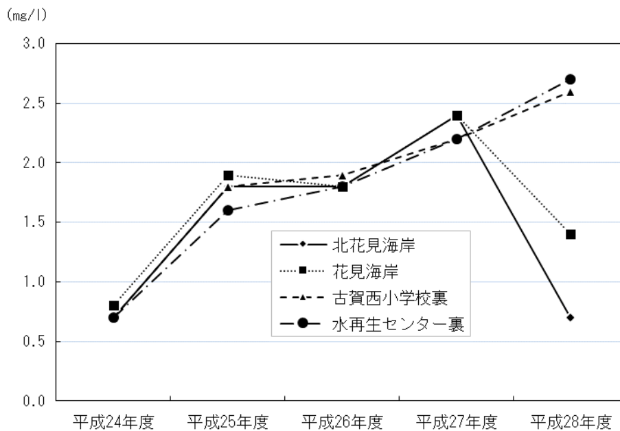
図 10 海水域水質調査結果（COD）
