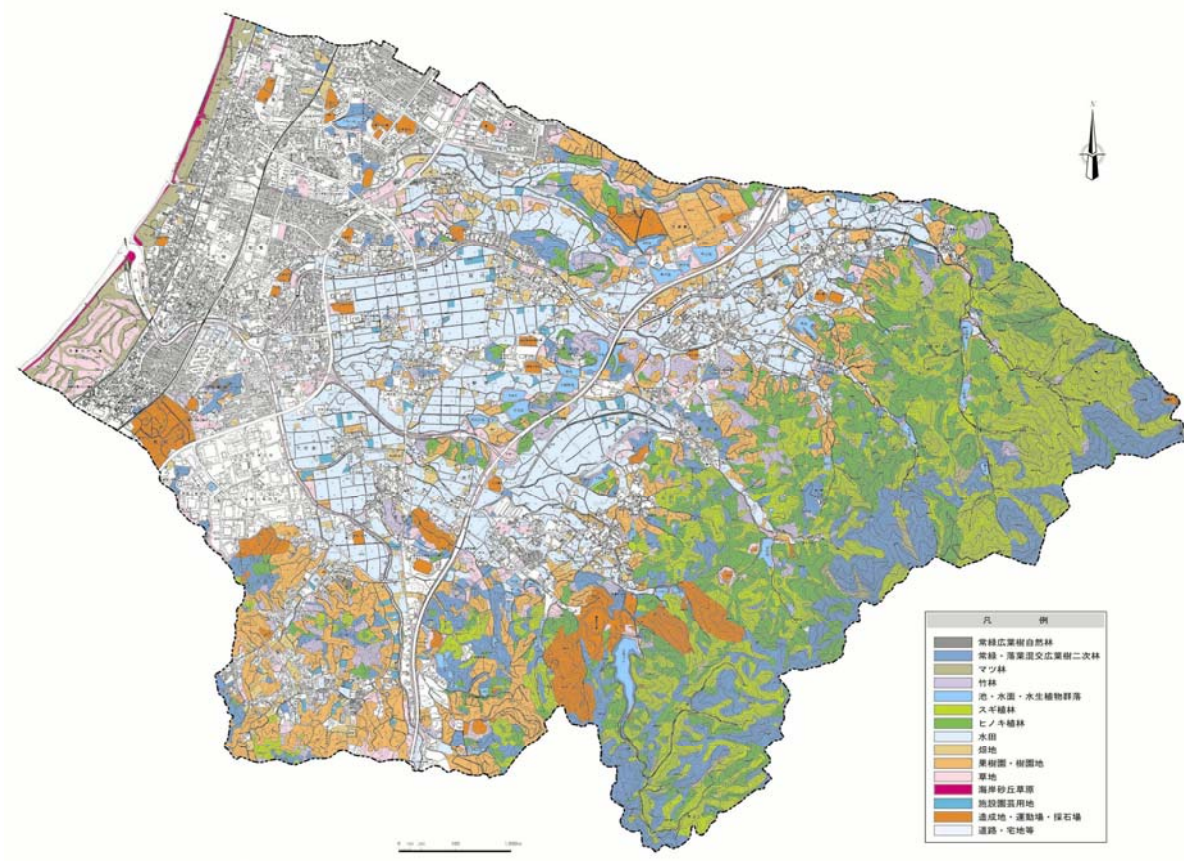
図 14 植生図
