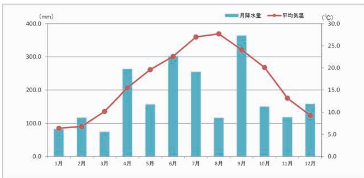
図2-4 平成28（2016）年 月別平均気温と降水量（資料：気象庁 HP 宗像観測所）
