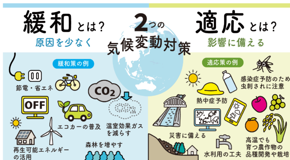
図 1-2 緩和と適応
