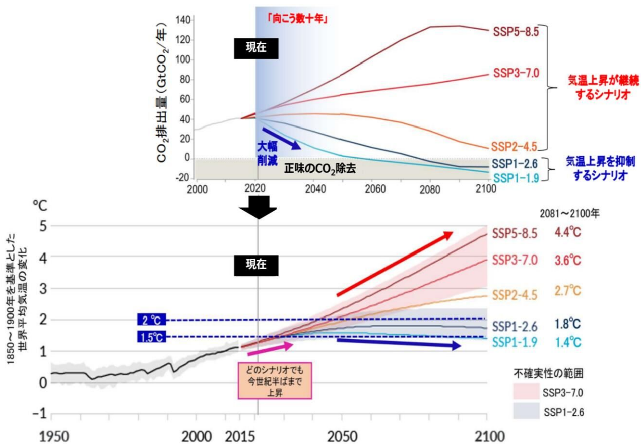
図 1-9 将来シナリオにおける CO 2 排出量と世界平均気温の変化
