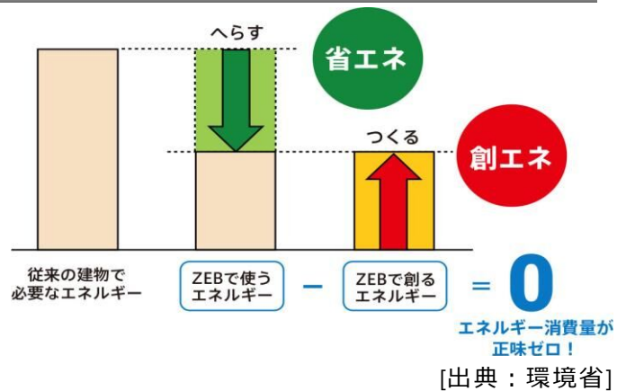
図 3-12 ZEB の考え方と定義
