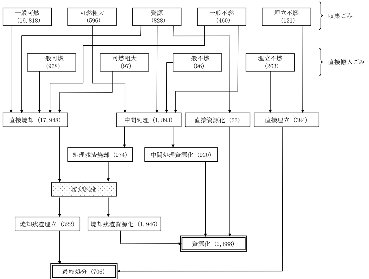
図 3 ごみ処理フロー図（平成 17 年度）
